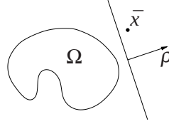
Figura 3.4: Hiperplano separador \rho^T x = \delta .
