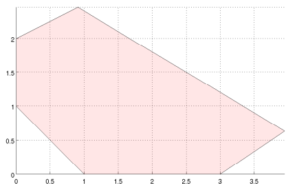
Figura 4.2: Região viável
