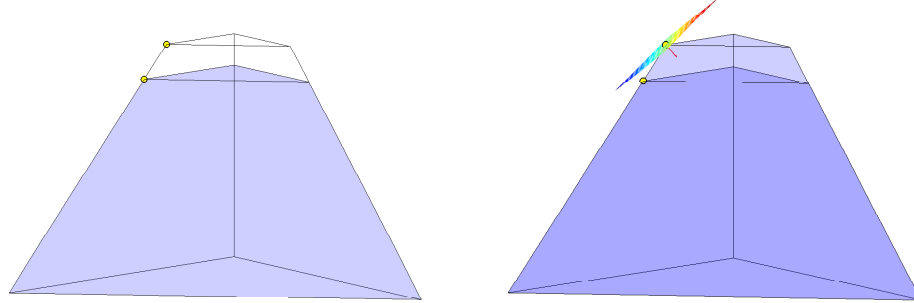
Figura 5.5: Problema à esquerda p_1 no nível 1
