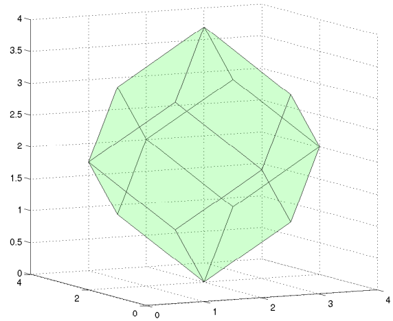
Figura 4.4: Região viável
