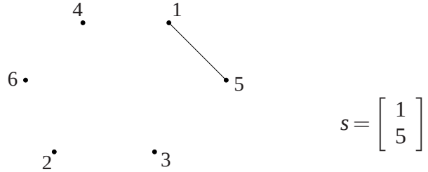
Figura 3.9: Construção da aresta
