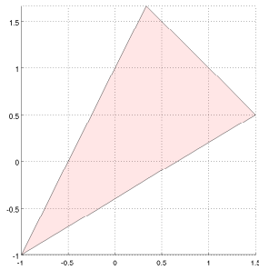
Figura 3.11: poliedro(A,b,2,'r')
