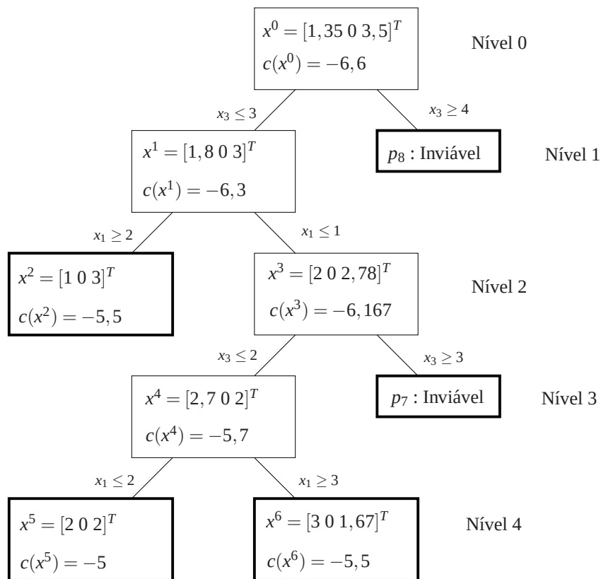
Figura 5.12: Árvore completa
